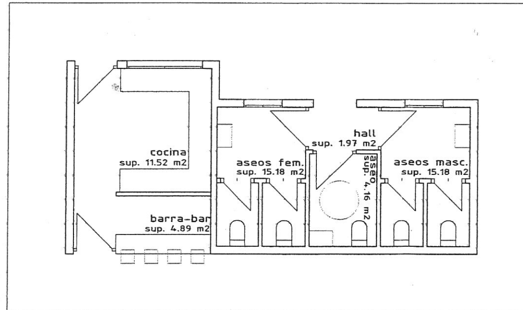
planta baja e_1.100
