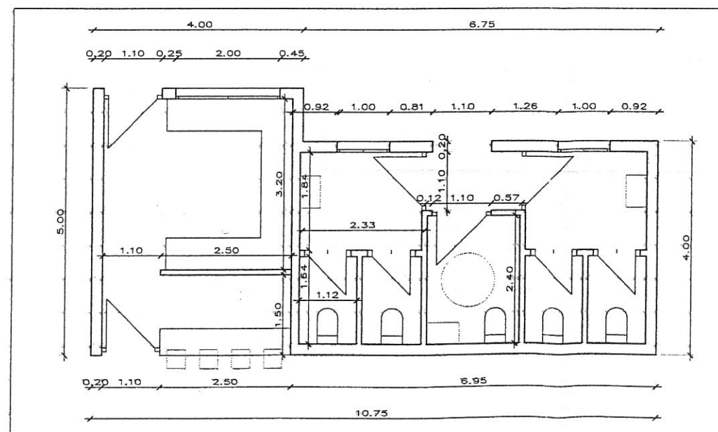
planta baja acotada e_1.100
