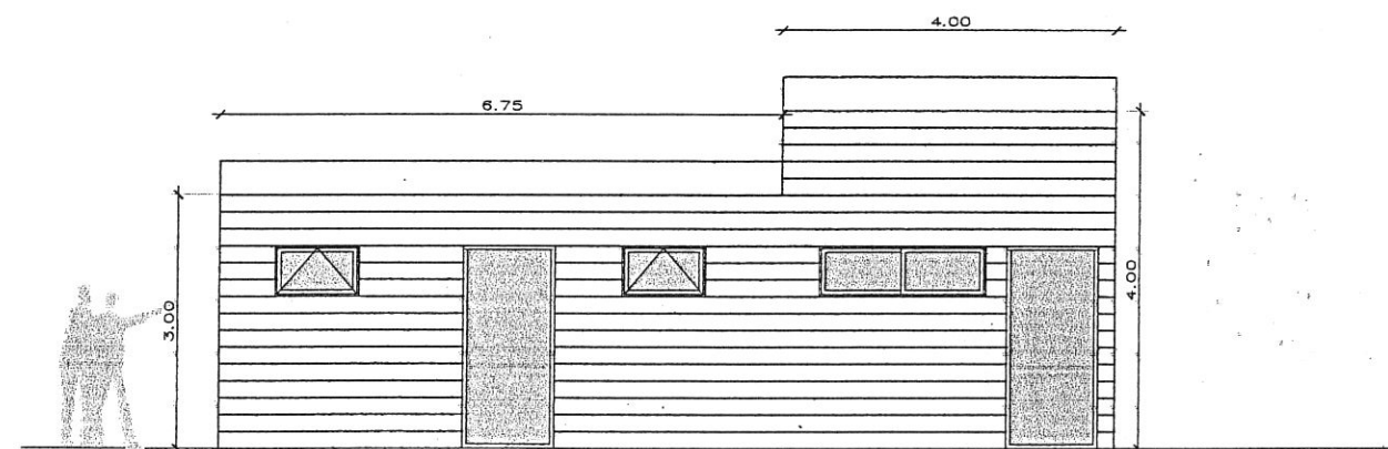
alzado norte e_1.100
