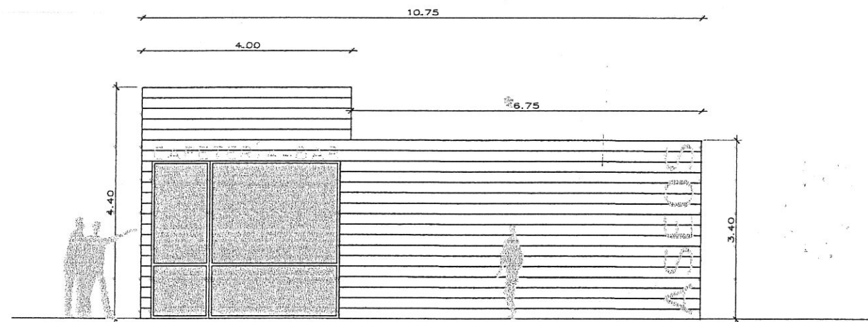
alzado sur e_1.100
